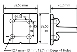
Drwg. B : HCCP - 4120 / HCCP - 4240
